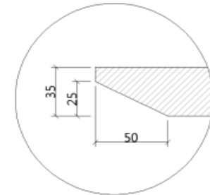
Wood veneer 35mm Inward bevel edge
